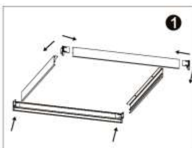
1. Assembler le cadre avec les 4 fixations d'angle
